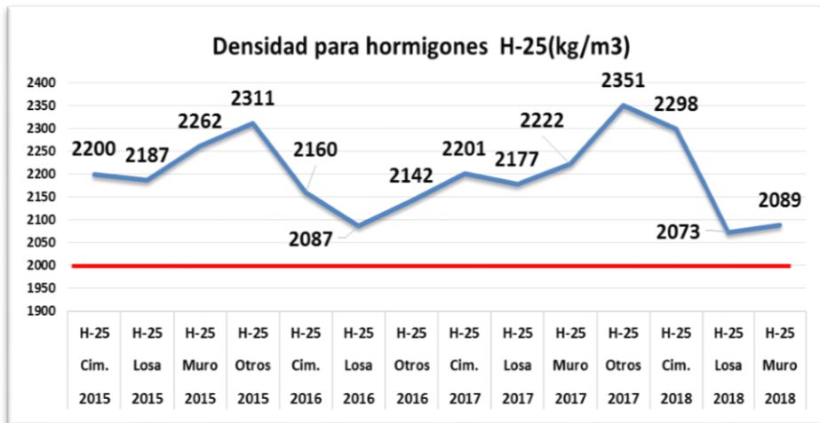
FIGURA No.7A: VALORES DE RESISTENCIAS A COMPRESIÓN, DENSIDADES Y POROSIDADES EFECTIVAS, ALCANZADOS EN EL PERIODO, EN HORMIGONES H-25. (FUENTE: ELABORACIÓN PROPIA)
