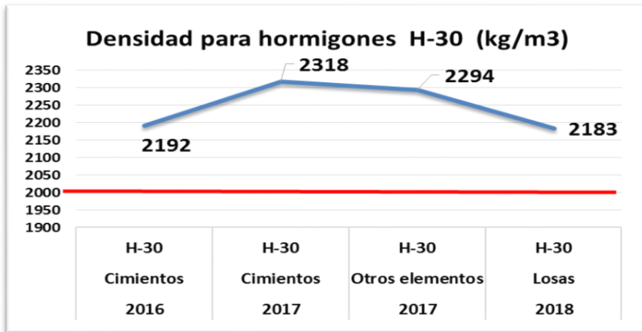
FIGURA No. 7B: VALORES DE RESISTENCIAS A COMPRESIÓN, DENSIDADES Y POROSIDADES EFECTIVAS, ALCANZADOS EN EL PERIODO, EN HORMIGONES H-30. (FUENTE: ELABORACIÓN PROPIA)
